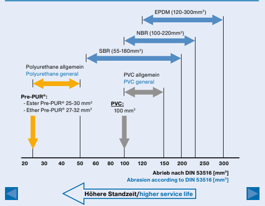
Bild 2/ Fig. 2: Abriebfestigkeit/Abrasion resistance
