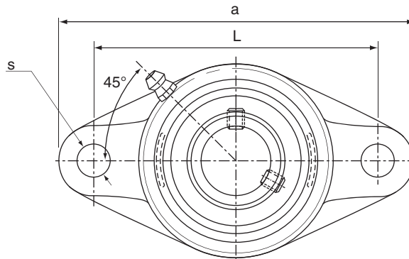
UCFL 200 Фланцевые узлы с 2 отверстиями
