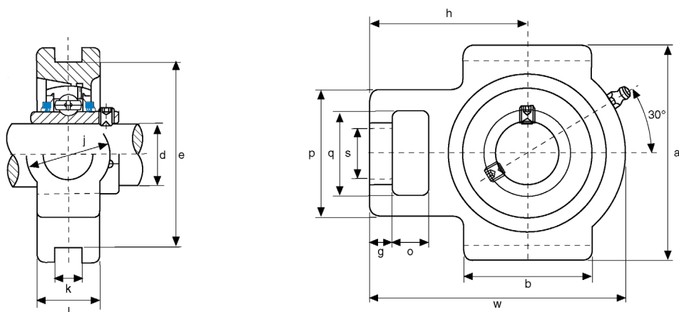
УСТ 200E Натяжные подшипниковые узлы
