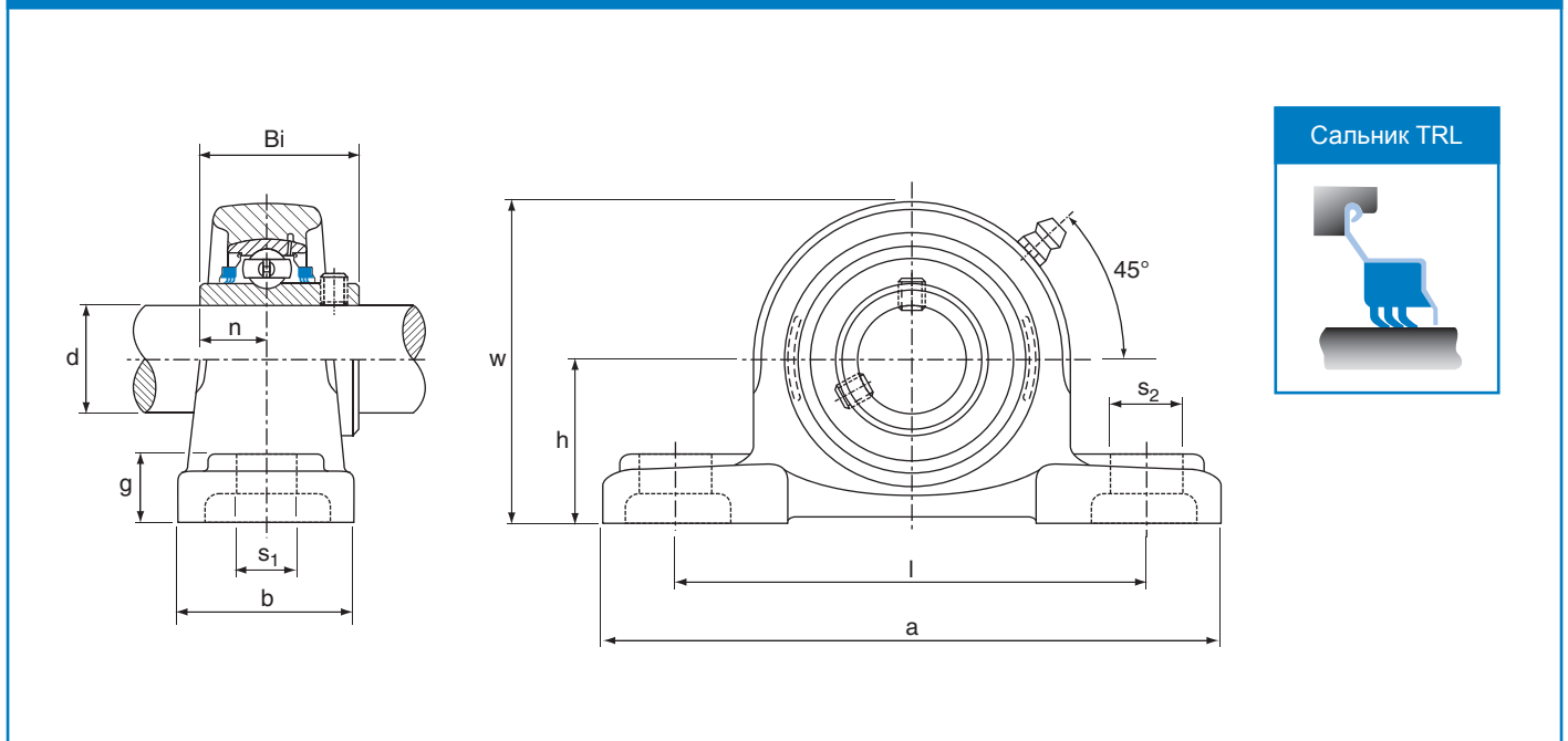
UCP 200 Корпусные подшипники
