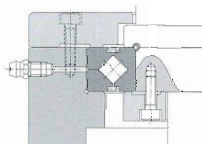
б. Вращение внутреннего кольца в шарнирном блоке (с установленными уплотнениями)
