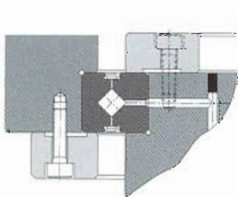
а. Вращение наружного кольца в шарнирном блоке: Пример установки тяжёлой детали после закрепления внутреннего и наружного колец с поперечными роликами
