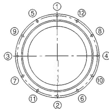
Рис. 1 Порядок затяжки
