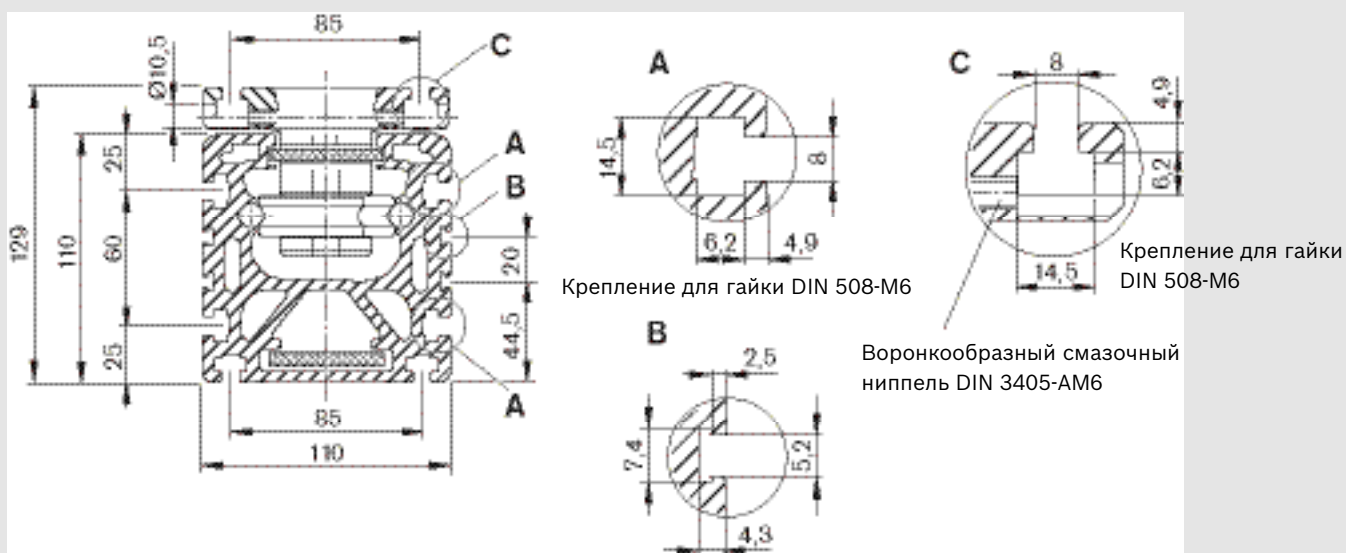
Крепление для кабельного канала
