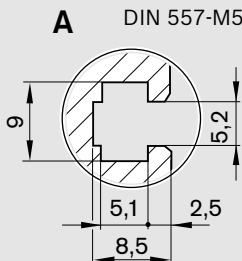
Крепление для гайки DIN 557-M5
