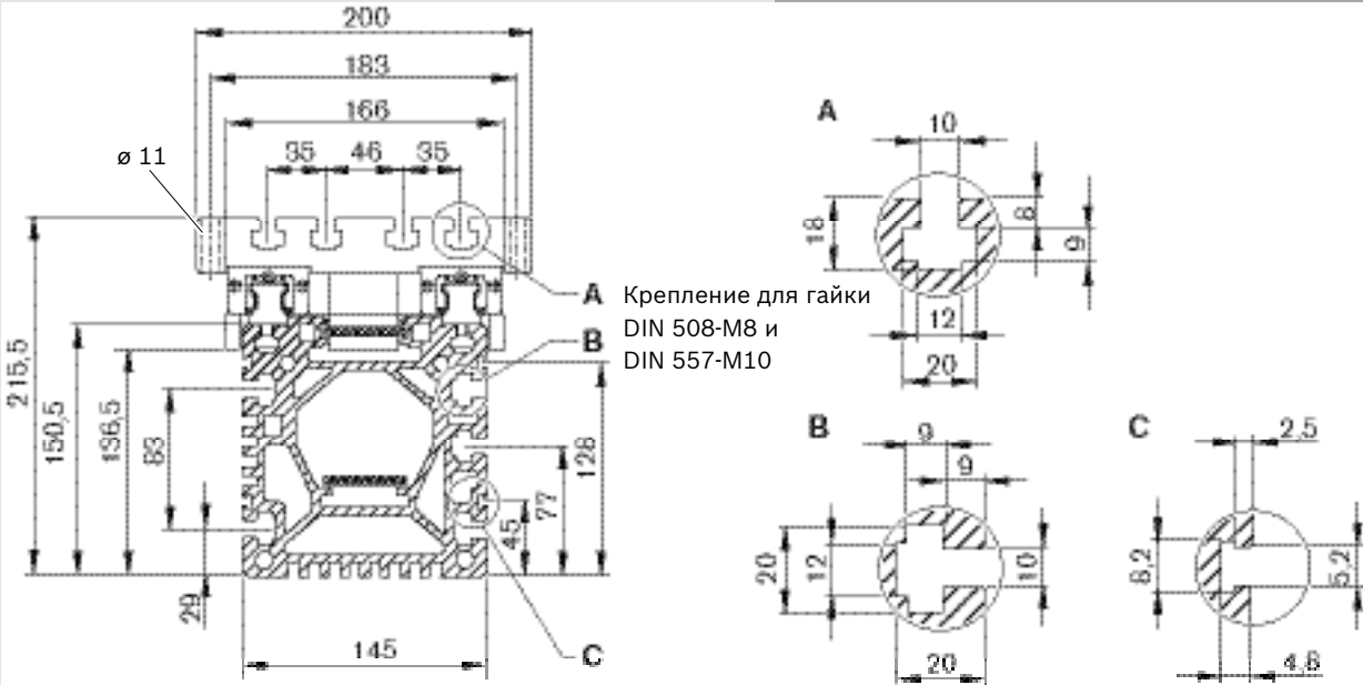
Крепление для кабельного канала
