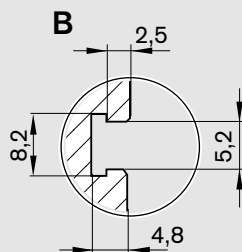
Крепление для кабельного канала
