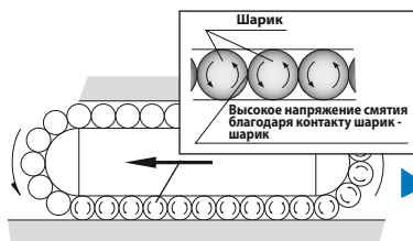
Стандартная конструкция
