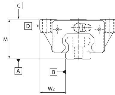
Деталь: мм
