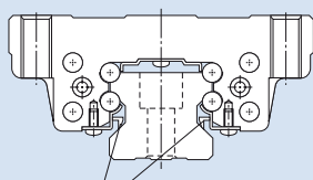
Боковое уплотнение
